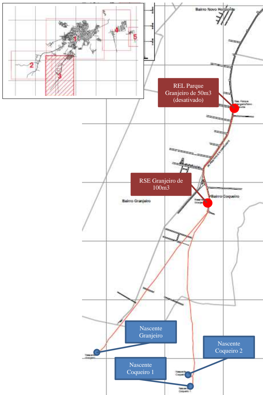
Figura 7.6 – Croqui do sistema de abastecimento de água da sede do Crato.
