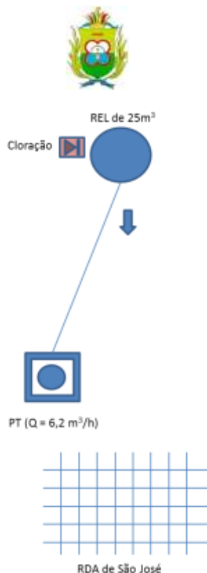
Figura 7.68 – Croqui do sistema de abastecimento de água da localidade de São José, no município do Crato, de responsabilidade do SISAR.
