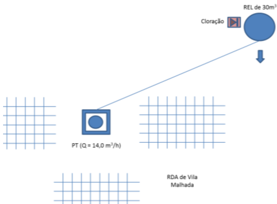
Figura 7.53 – Croqui do sistema de abastecimento de água da localidade de Vila Malhada, no município do Crato, de responsabilidade do SISAR.
