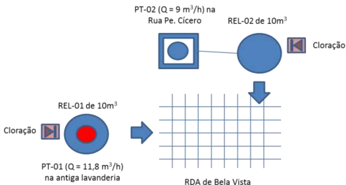
Figura 7.35 – Croqui do sistema de abastecimento de água do distrito de Bela Vista, no município do Crato, de responsabilidade da SAAEC.
