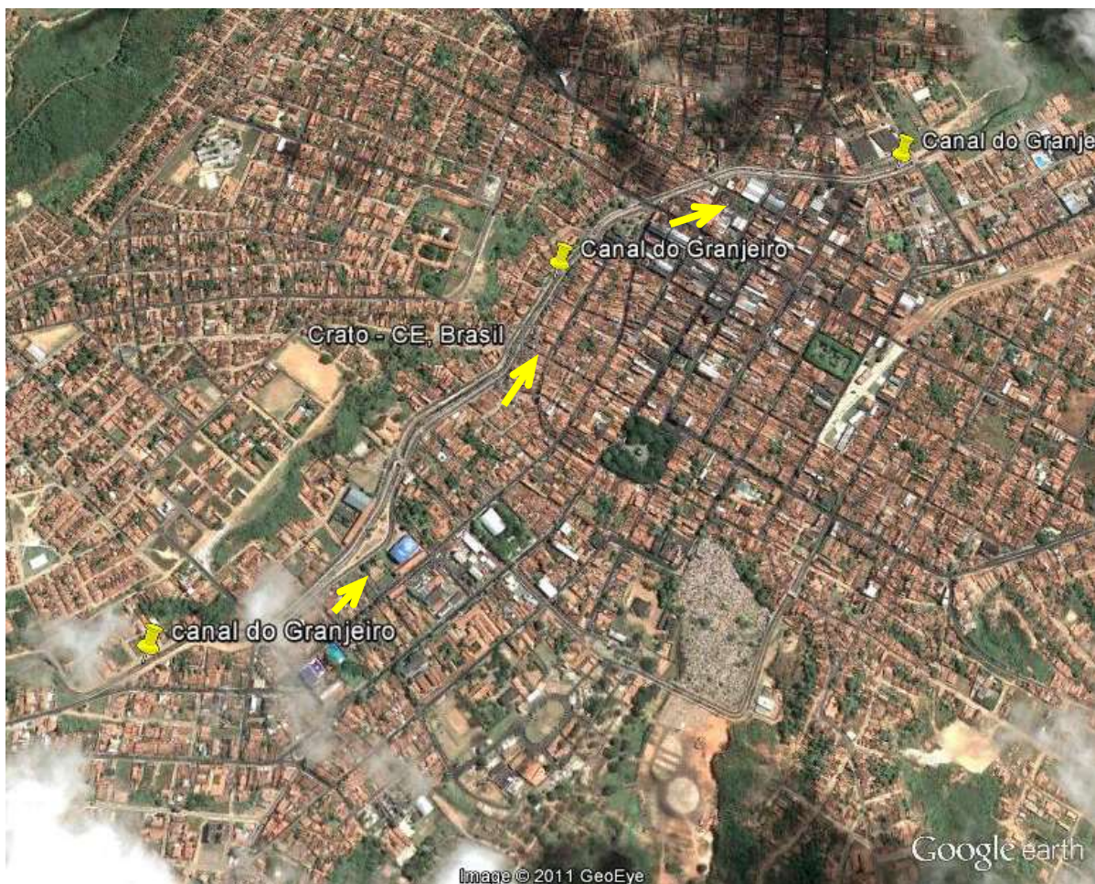
Figura 7.144 – Macrodrenagem da cidade do Crato, com destaque para o início e o fim do trecho canalizado do rio Granjeiro.
