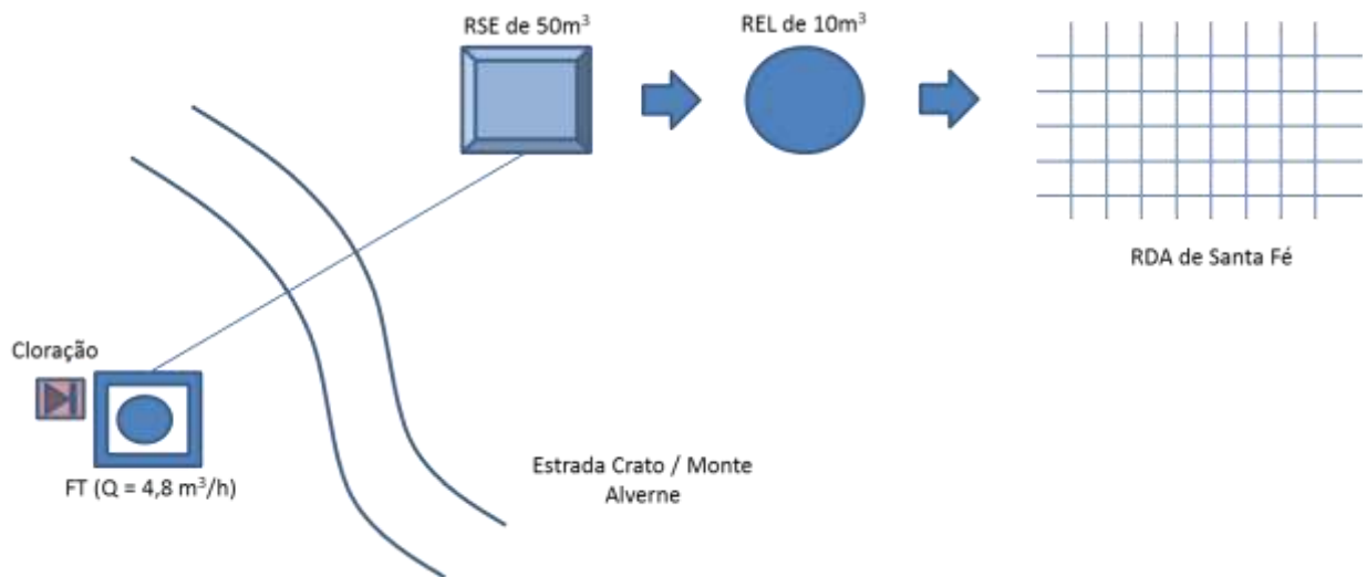
Figura 7.40 – Croqui do sistema de abastecimento de água do distrito de Santa Fé, no município do Crato, de responsabilidade da SAAEC.
