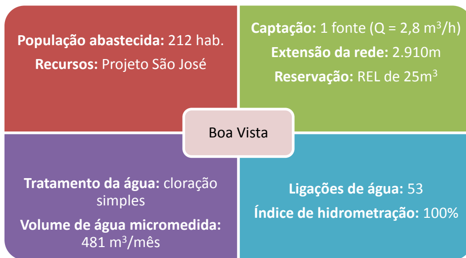
Figura 7.78 –Dados sobre o abastecimento de água da localidade de Boa Vista, no município do Crato, de responsabilidade do SISAR.
