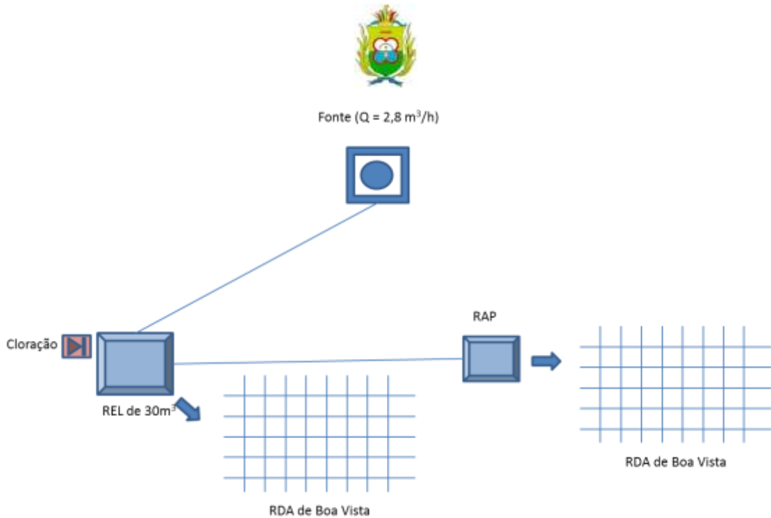
Figura 7.77 – Croqui do sistema de abastecimento de água da localidade de Boa Vista, no município do Crato, de responsabilidade do SISAR.
