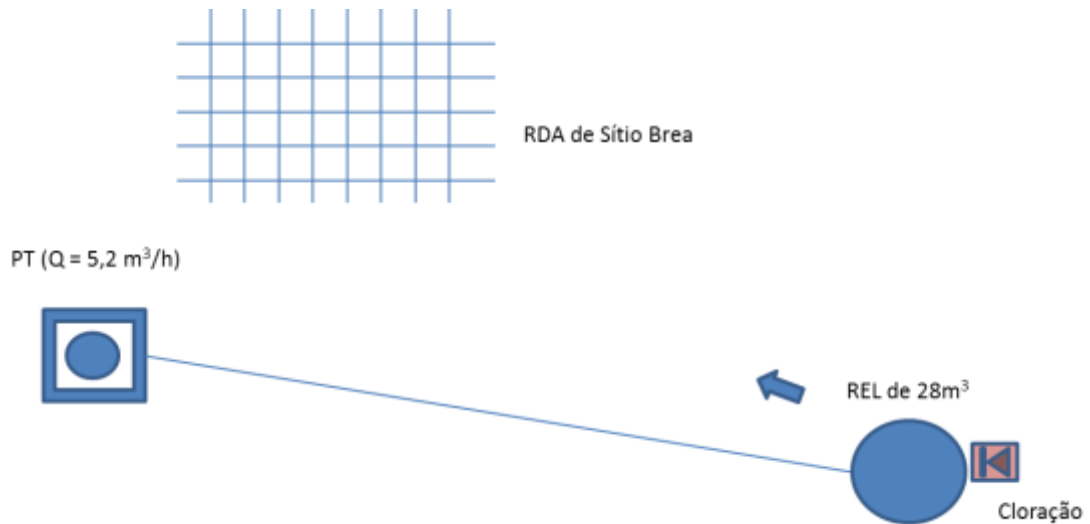
Figura 7.98 – Croqui do sistema de abastecimento de água da localidade de Sítio Brea, no município do Crato, de responsabilidade do SISAR.
