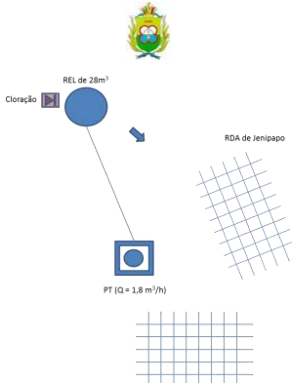
Figura 7.80 – Croqui do sistema de abastecimento de água da localidade de Jenipapo, no município do Crato, de responsabilidade do SISAR.
