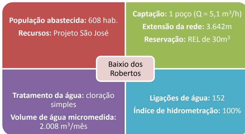
Figura 7.84 —Dados sobre o abastecimento de água da localidade de Baixo dos Robertos, no município do Crato, de responsabilidade do SISAR.
