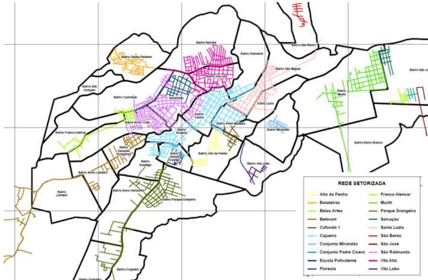
Figura 7.1 – Setorização do sistema de abastecimento de água da sede do Crato.
