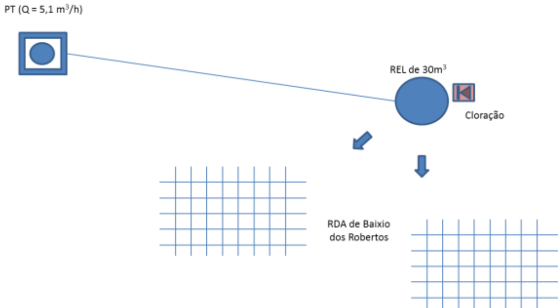
Figura 7.83 – Croqui do sistema de abastecimento de água da localidade de Baixo dos Robertos, no município do Crato, de responsabilidade do SISAR.
