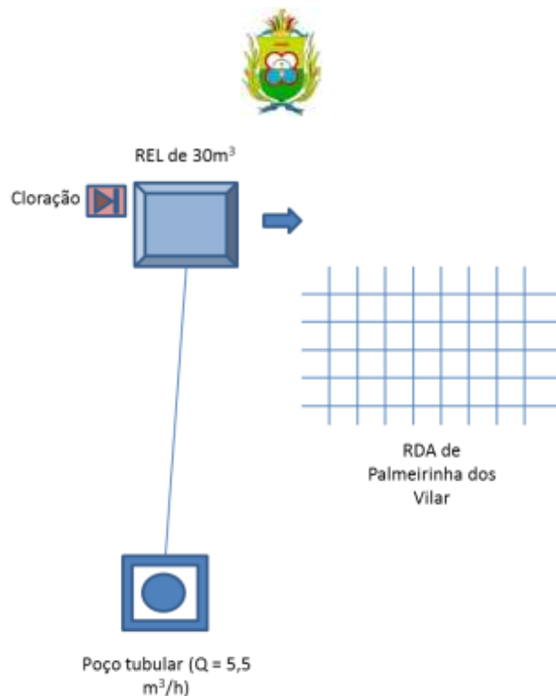
Figura 7.74 – Croqui do sistema de abastecimento de água da localidade de Palmeirinha dos Vilar, no município do Crato, de responsabilidade do SISAR. Fonte: Consórcio DGH-Cariri (2012).
