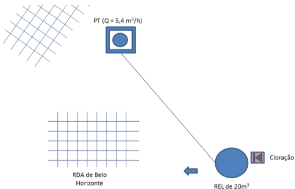
Figura 7.71 – Croqui do sistema de abastecimento de água da localidade de Belo Horizonte, no município do Crato, de responsabilidade do SISAR.
