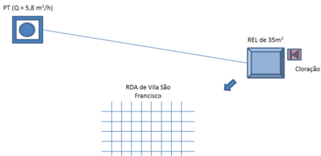
Figura 7.86 – Croqui do sistema de abastecimento de água da localidade de Vila São Francisco, no município do Crato, de responsabilidade do SISAR.
