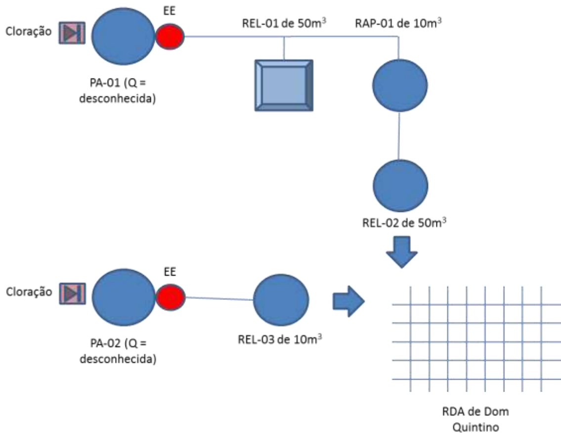
Figura 7.30 – Croqui do sistema de abastecimento de água do distrito de Dom Quintino, no município do Crato, de responsabilidade da SAAEC.
