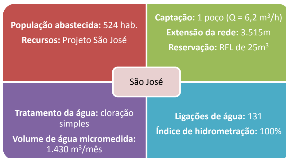
Figura 7.69 –Dados sobre o abastecimento de água da localidade de São José, no município do Crato, de responsabilidade do SISAR.
