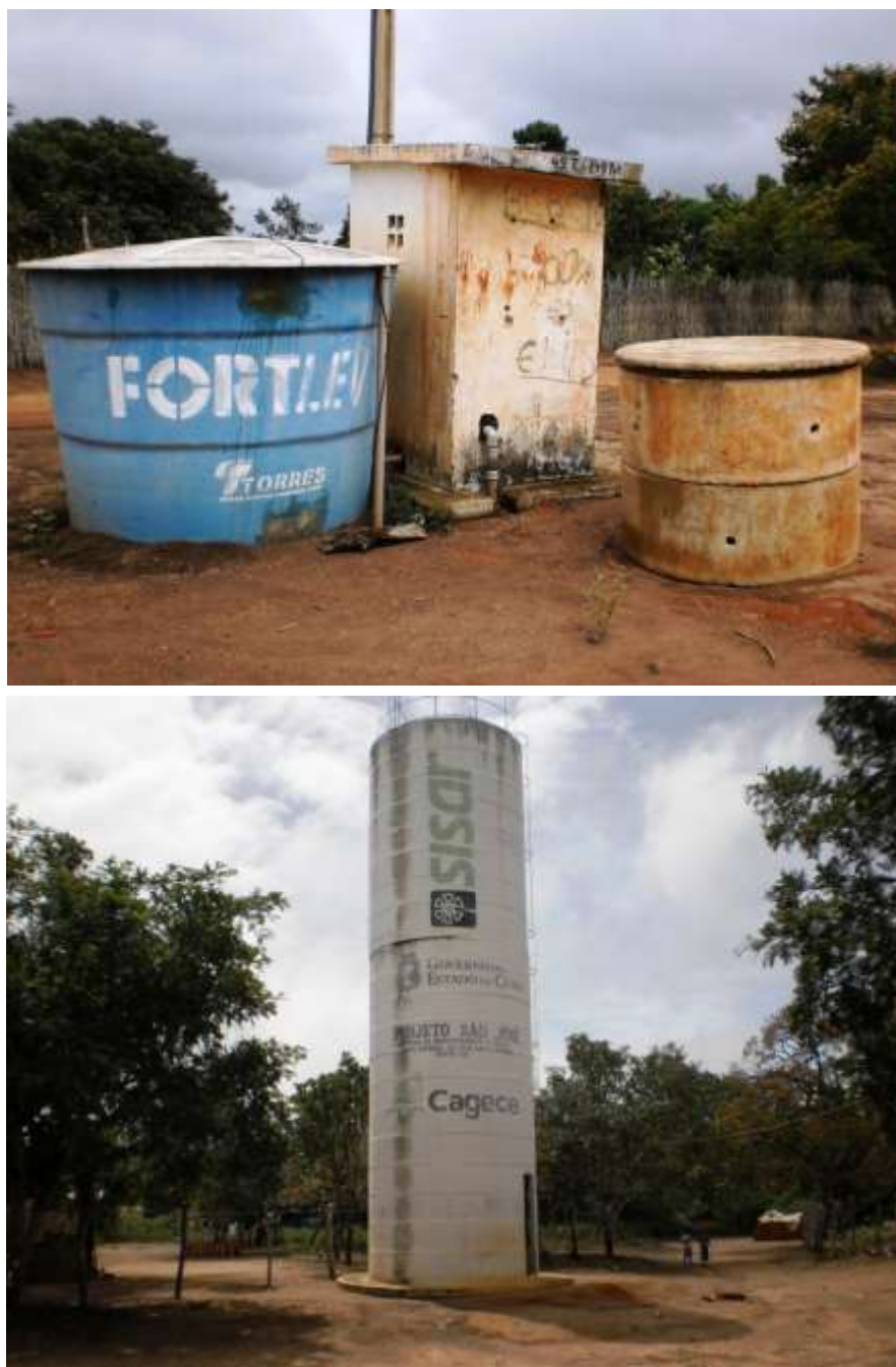
Figura 7.91 – Vista do poço tubular ( Q = 5,1 \text{ m}^3/\text{h} ) e REL de 25 \text{ m}^3 que fazem parte do sistema da localidade de Santo Antônio, município do Crato, de responsabilidade do SISAR.
