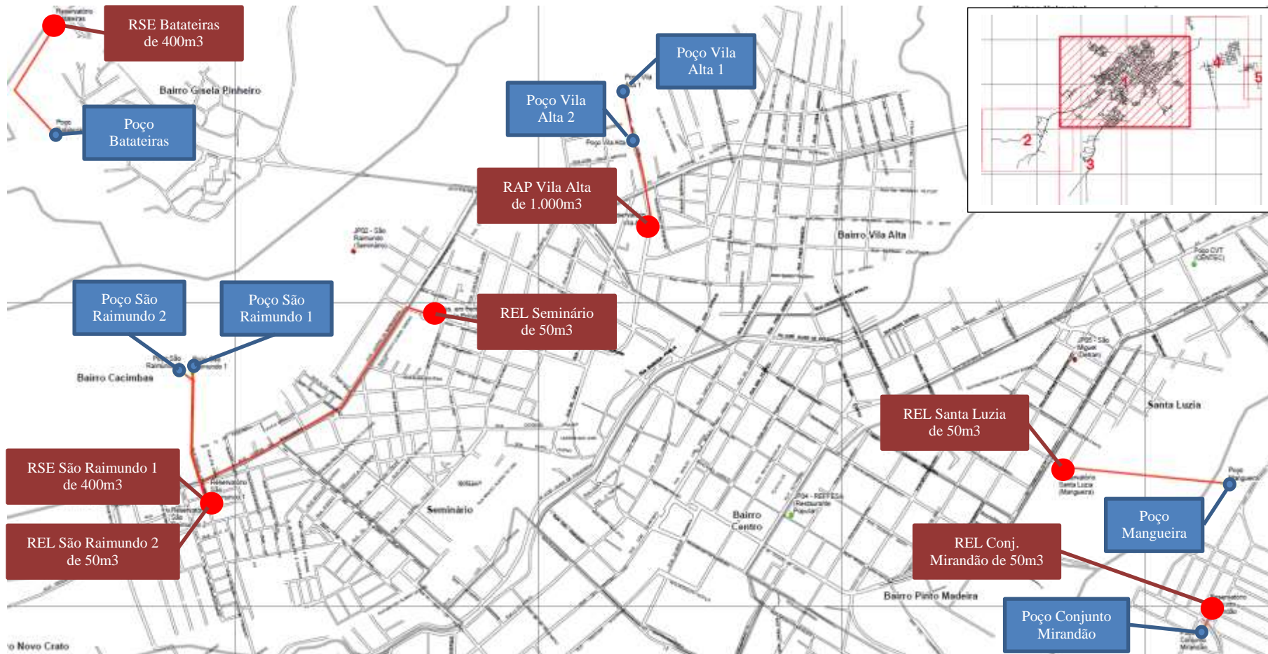
Figura 7.2 – Croqui do sistema de abastecimento de água da sede do Crato.
