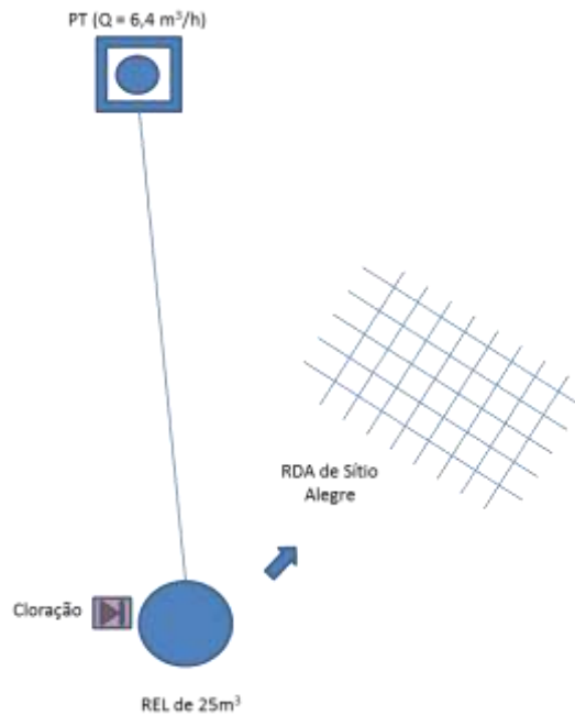
Figura 7.59 – Croqui do sistema de abastecimento de água da localidade de Sítio Alegre, no município do Crato, de responsabilidade do SISAR.
