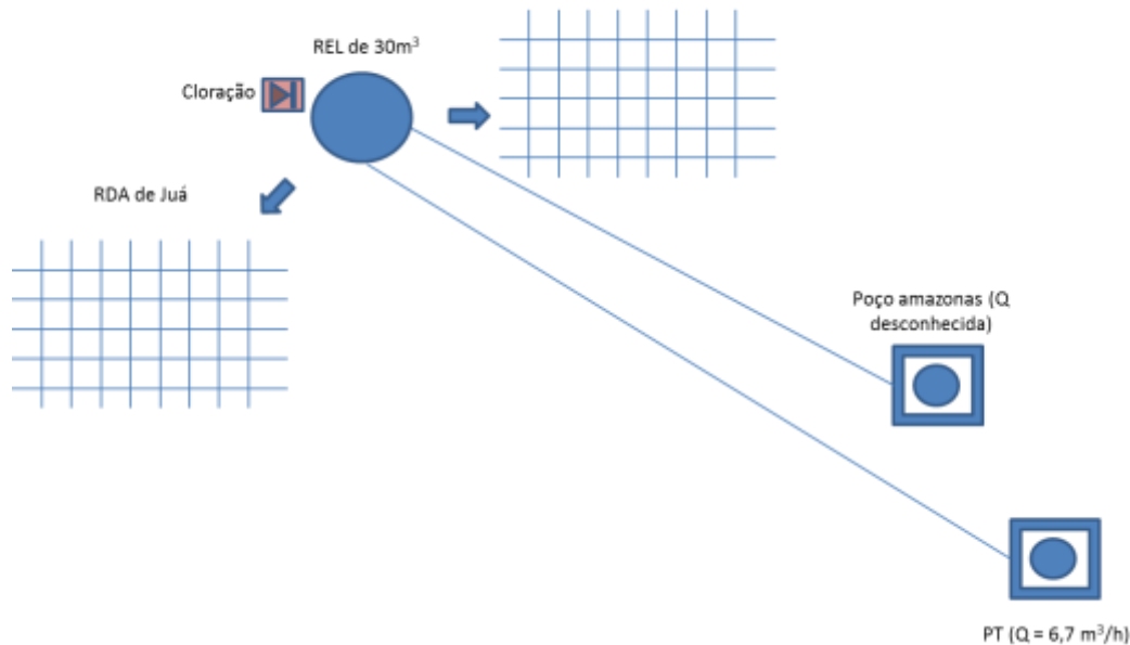
Figura 7.47 – Croqui do sistema de abastecimento de água da localidade de Juá, no município do Crato, de responsabilidade do SISAR.
