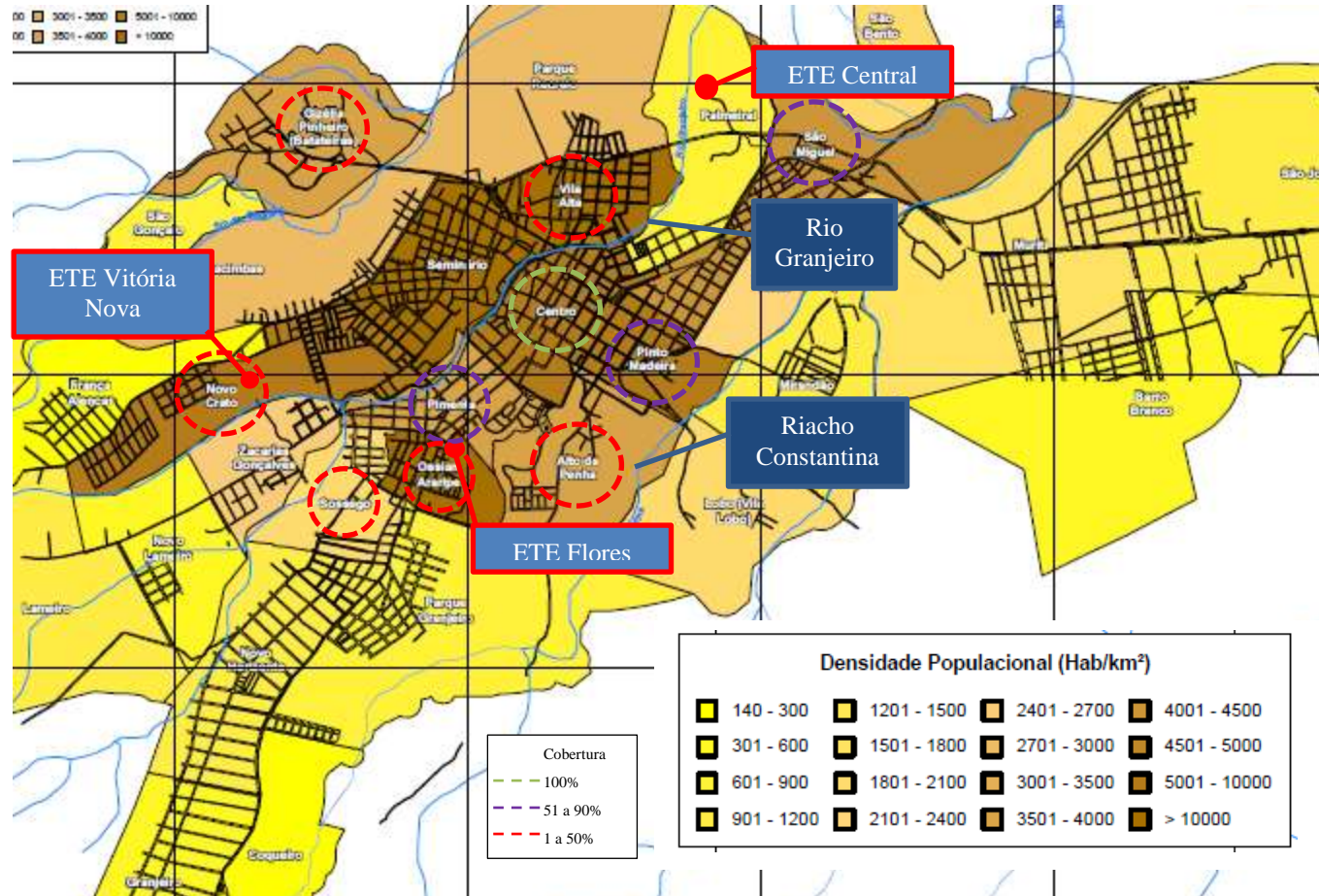
Figura 7.104 – Croqui do sistema de esgotamento sanitário da sede do Crato, de responsabilidade da SAAEC.
