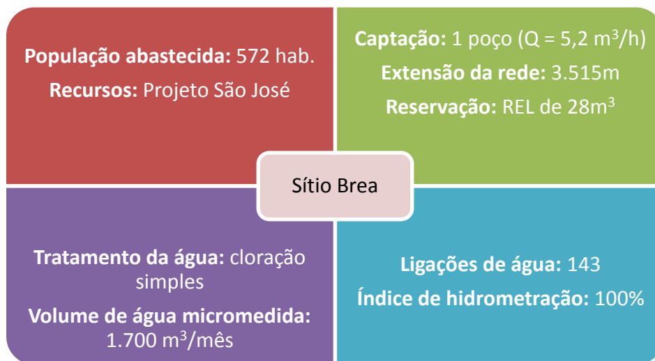
Figura 7.99 –Dados sobre o abastecimento de água da localidade de Sítio Brea, no município do Crato, de responsabilidade do SISAR.
