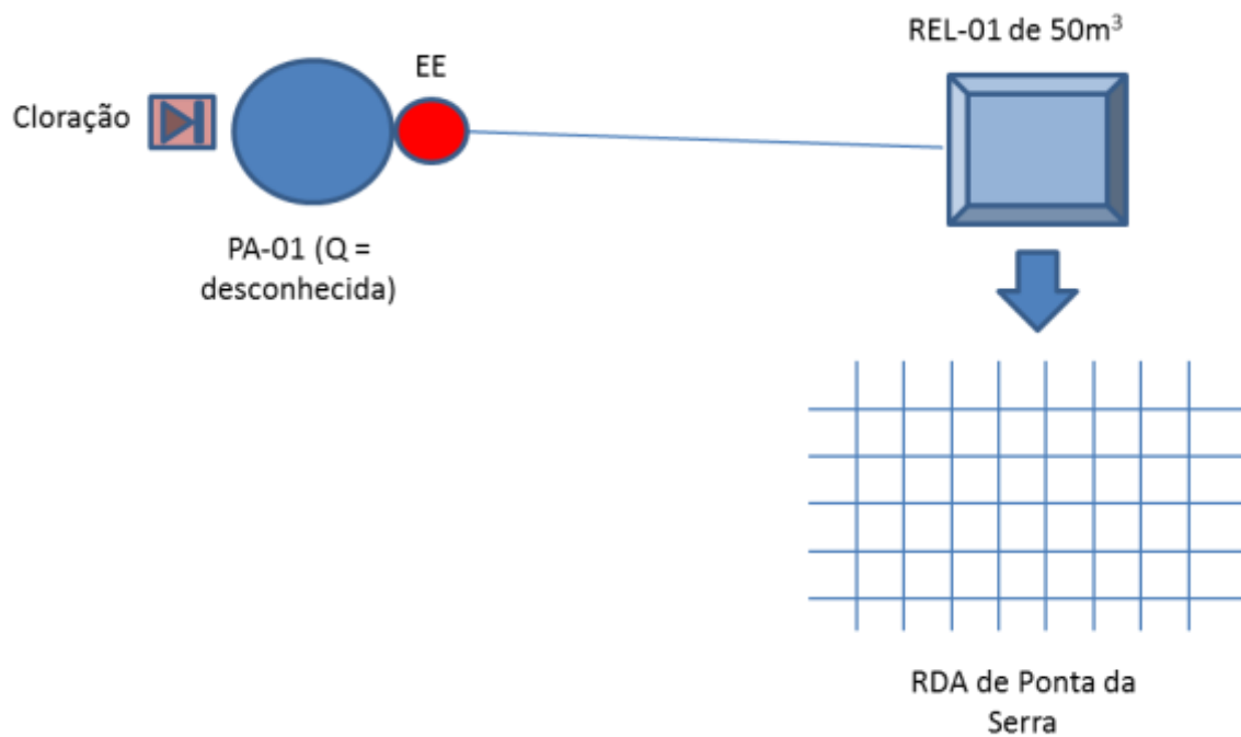
Figura 7.37 – Croqui do sistema de abastecimento de água do distrito de Ponta da Serra, no município do Crato, de responsabilidade da SAAEC.
