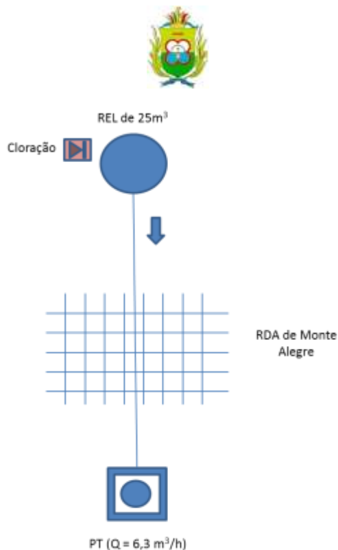
Figura 7.50 – Croqui do sistema de abastecimento de água da localidade de Monte Alegre, no município do Crato, de responsabilidade do SISAR.
