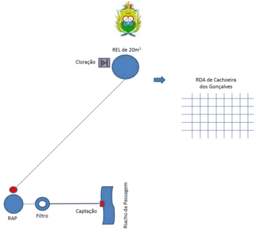
Figura 7.95 – Croqui do sistema de abastecimento de água da localidade de Cachoeira dos Gonçalves, no município do Crato, de responsabilidade do SISAR.
