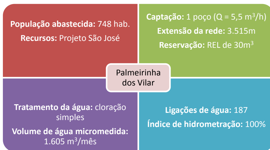
Figura 7.75 –Dados sobre o abastecimento de água da localidade de Palmeirinha dos Vilar, no município do Crato, de responsabilidade do SISAR. Fonte: Consórcio DGH-Cariri (2012).
