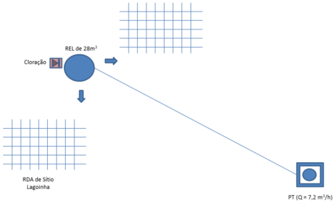
Figura 7.56 – Croqui do sistema de abastecimento de água da localidade de Lagoinha, no município do Crato, de responsabilidade do SISAR.
