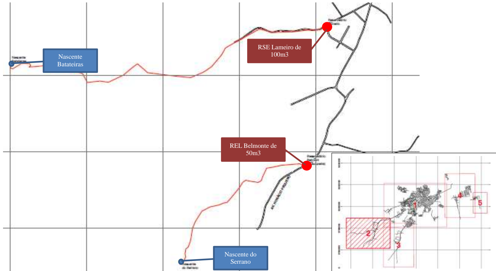
Figura 7.5 – Croqui do sistema de abastecimento de água da sede do Crato.
