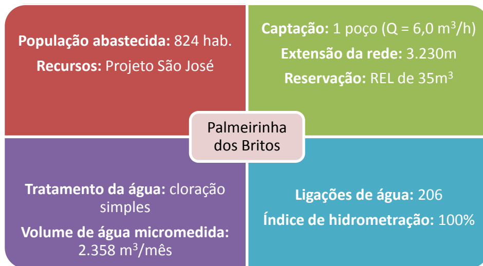
Figura 7.63 –Dados sobre o abastecimento de água da localidade de Palmeirinha dos Britos, no município do Crato, de responsabilidade do SISAR. Fonte: Consórcio DGH-Cariri (2012).
