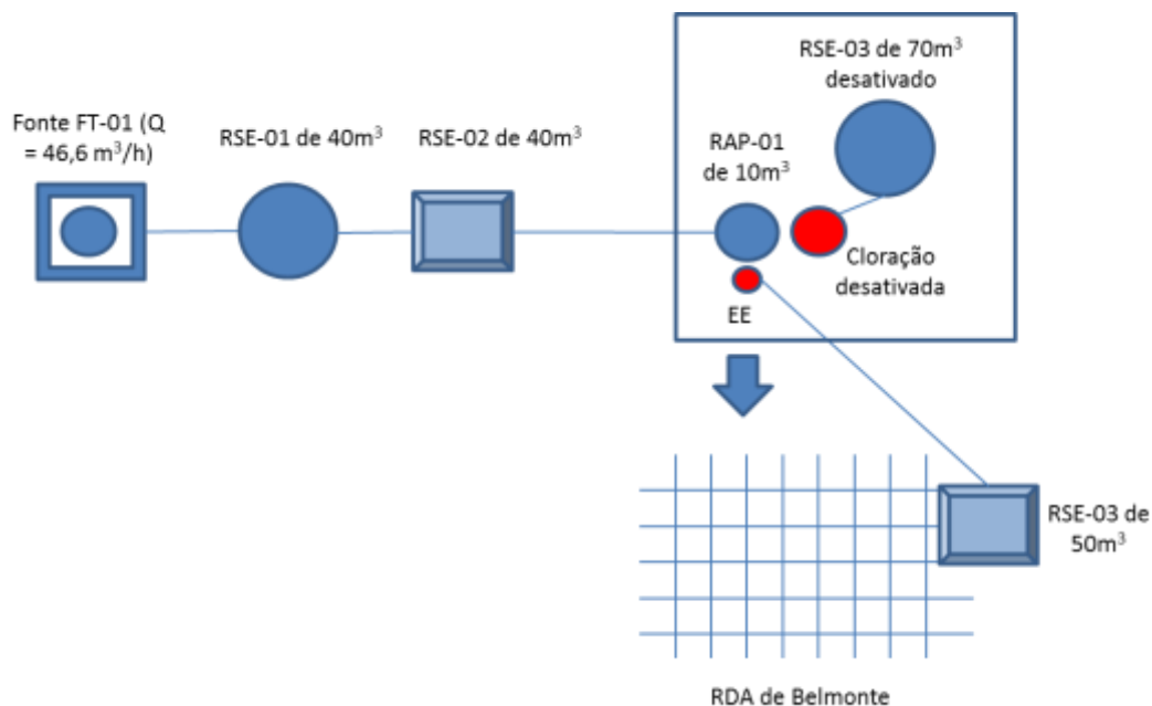
Figura 7.25 – Croqui do sistema de abastecimento de água do distrito de Belmonte, no município do Crato, de responsabilidade da SAAEC.
