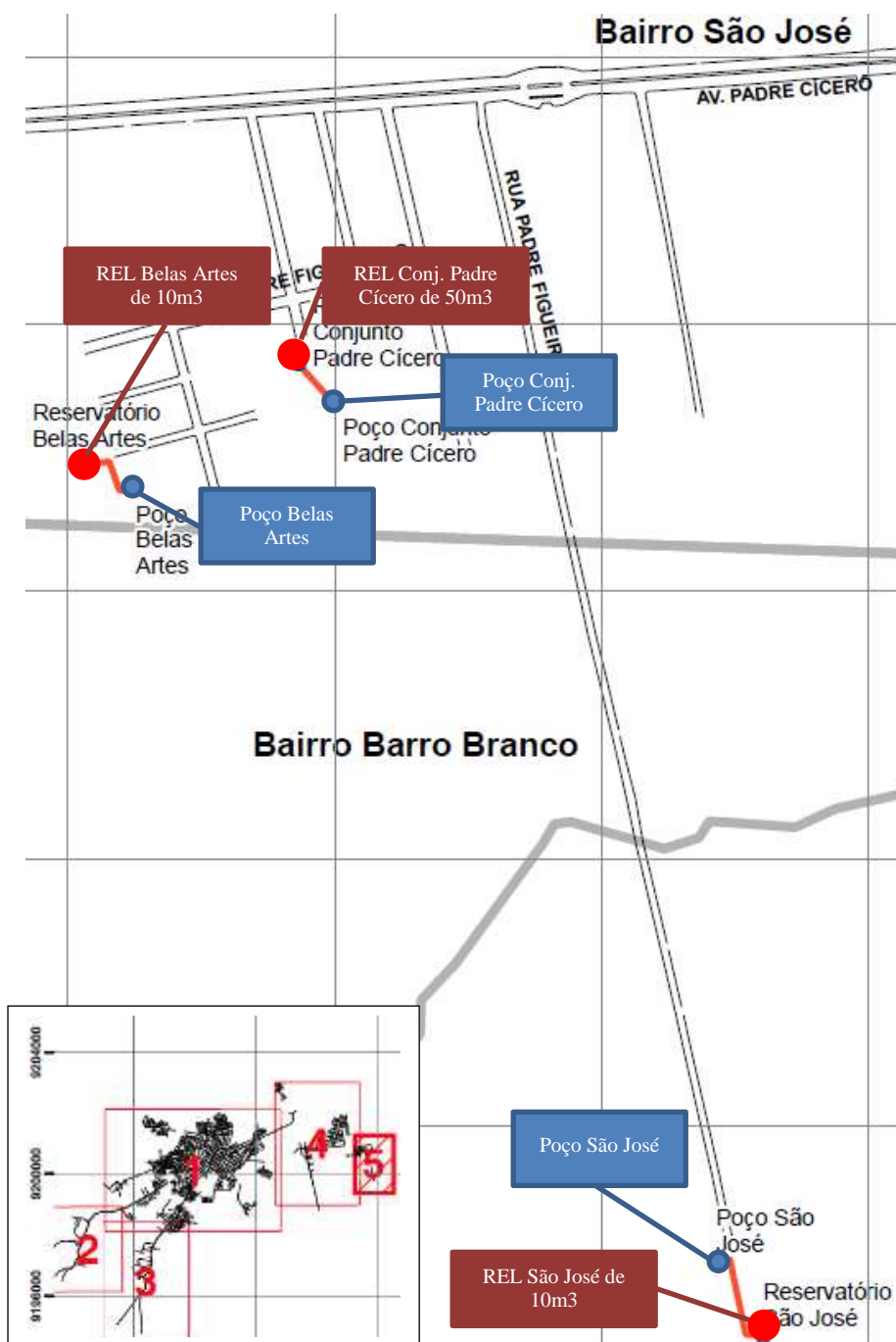
Figura 7.8 – Croqui do sistema de abastecimento de água da sede do Crato.
