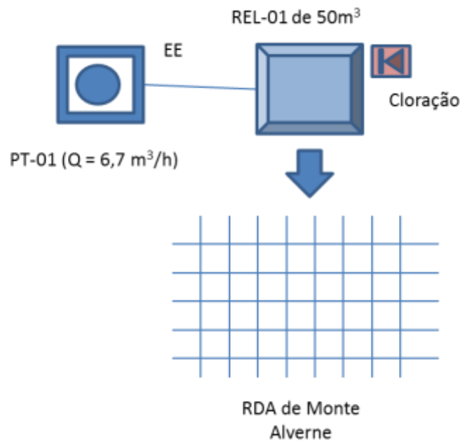
Figura 7.33 – Croqui do sistema de abastecimento de água do distrito de Monte Alverne, no município do Crato, de responsabilidade da SAAEC.
