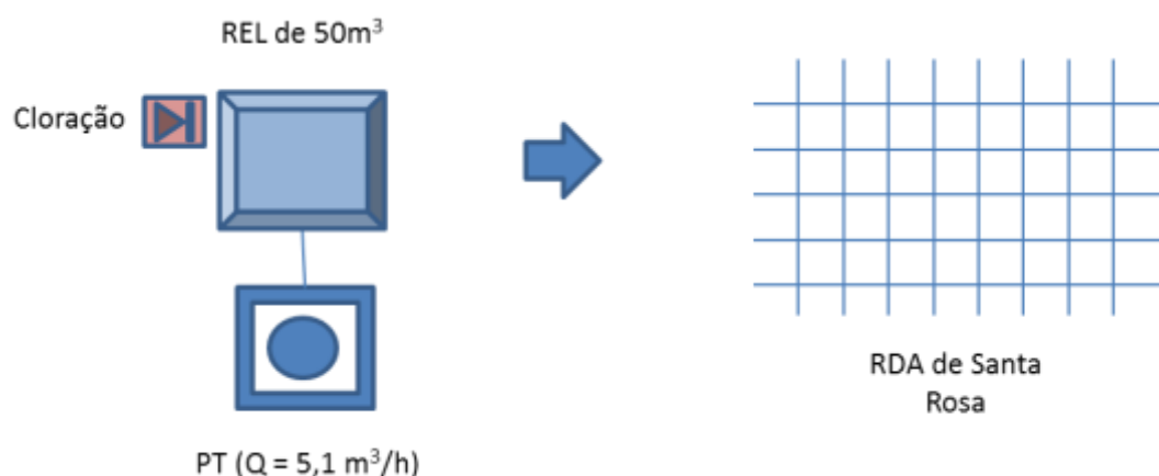
Figura 7.42 – Croqui do sistema de abastecimento de água do distrito de Santa Rosa, no município do Crato, de responsabilidade da SAAEC.
