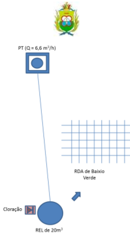
Figura 7.65 – Croqui do sistema de abastecimento de água da localidade de Baixo Verde, no município do Crato, de responsabilidade do SISAR.
