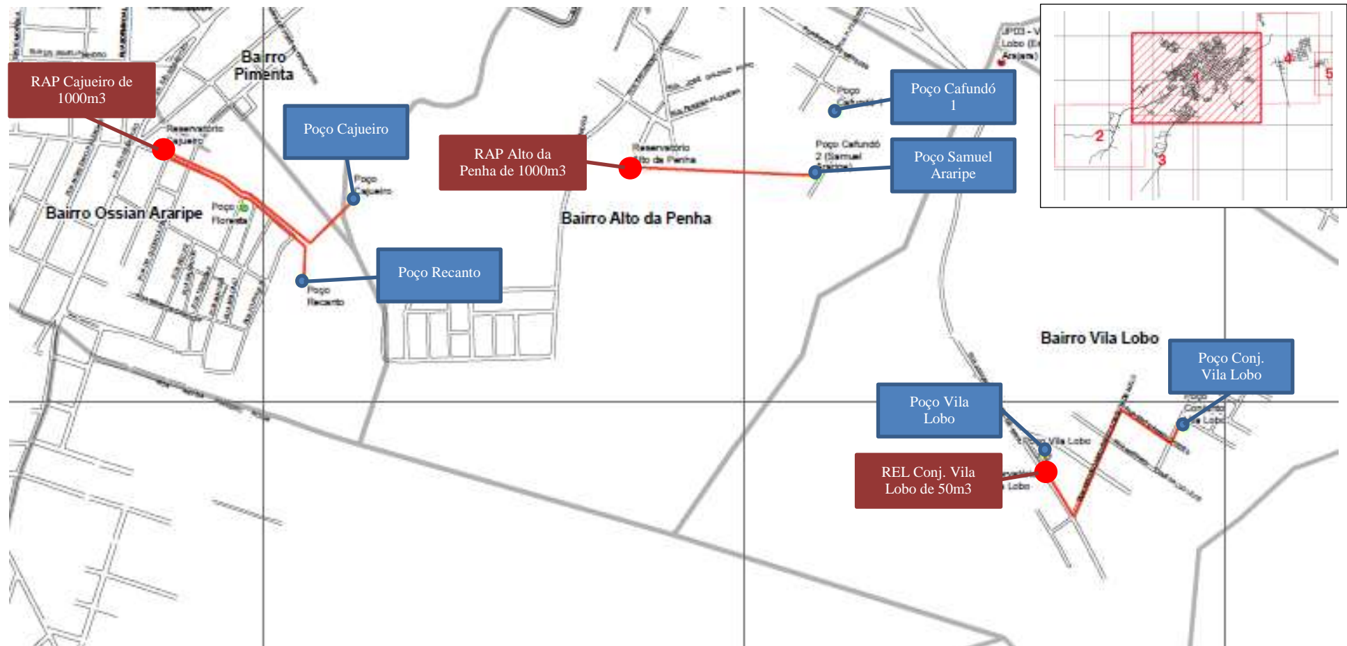
Figura 7.4 – Croqui do sistema de abastecimento de água da sede do Crato.
